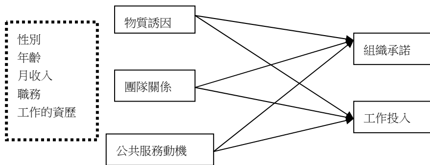
圖 1 研究架構圖
